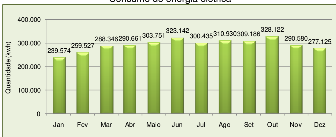
GRÁFICO 183 Histórico do consumo de energia elétrica
